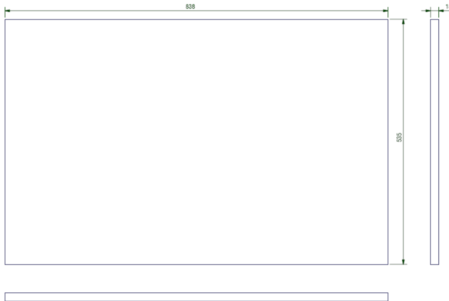
Vandfast krydsfiner montageplade Triax varenummer 232463 Der kan anvendes 1 eller 2 stk. (838x535x18 mm)
